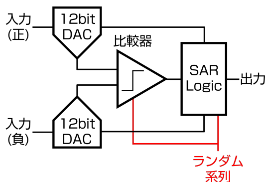
図1：設計した回路のブロック図
