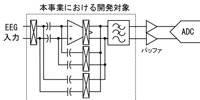
図 1: 脳波計測デバイスにおけるアナログフロントエンド
